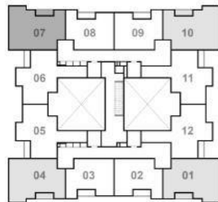
Pavimento tipo - Torre 2 - Final 07
